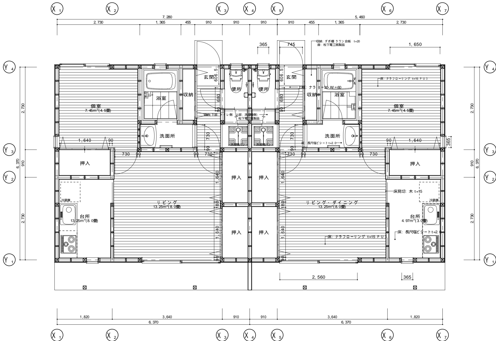
平面詳細図 scale: 1/50
