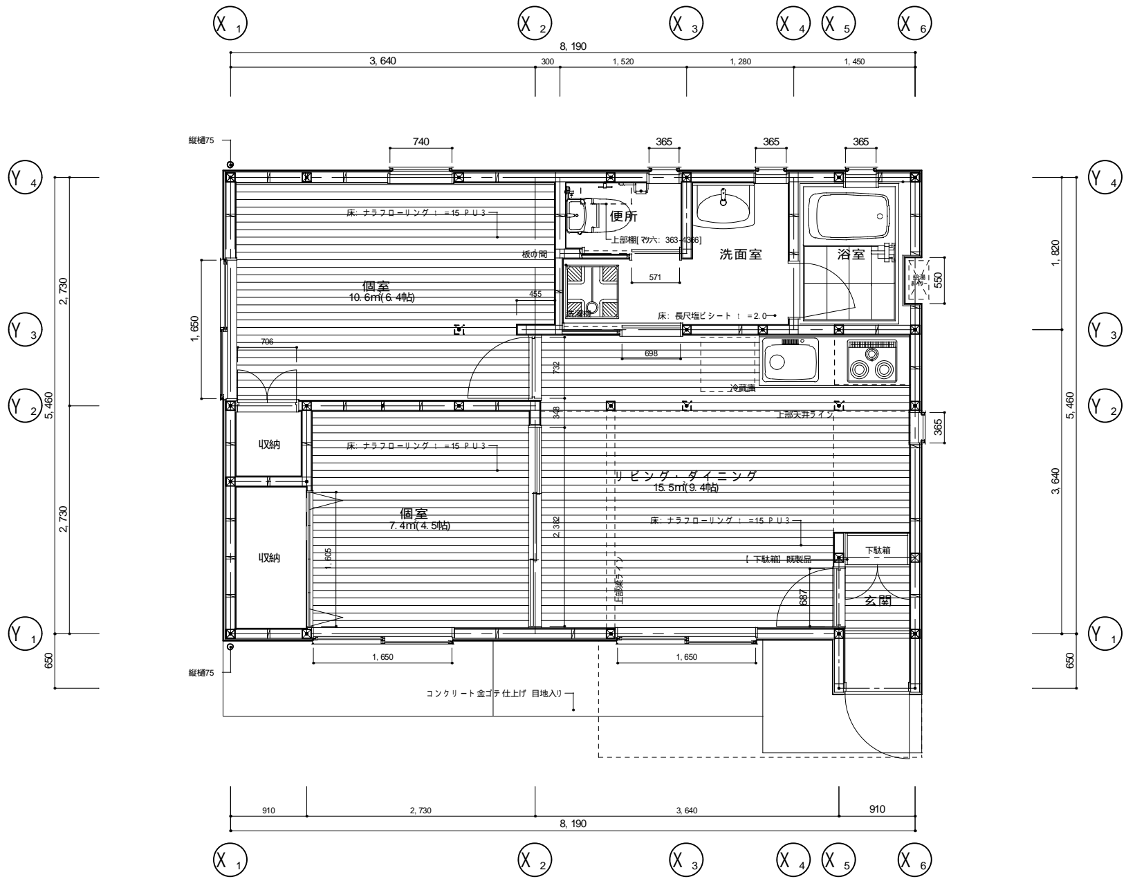
平面詳細図 scale: 1/50
